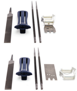
FEILENKIT 579 65 36-01
